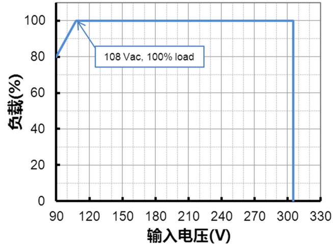
降额曲线
